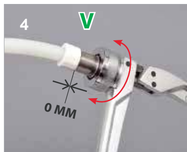
4 Расширение трубы (2). Шаг за шагом, проворачивая инструмент, перемещать далее трубу по расширительной насадке до упора. Поворот инструмента обязателен для равномерного расширения - правильного монтажа.
