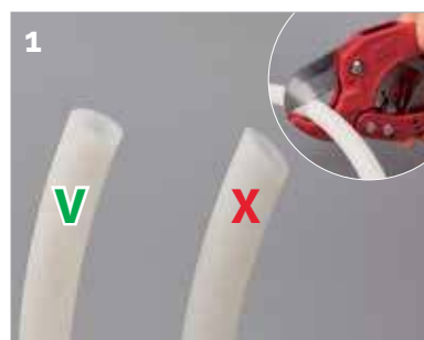
1 Резка трубы. Отрезать трубу перпендикулярно оси, не допуская ее деформирования.
